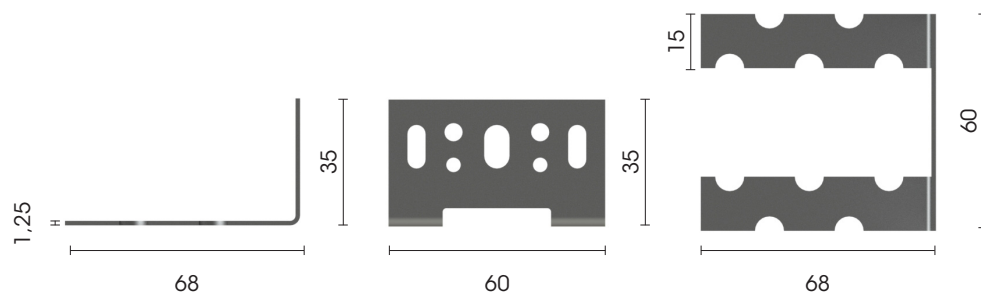
Wandanker
