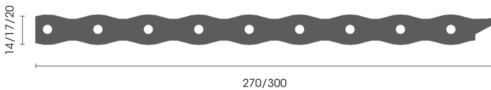
Lijmkoppelstrip Novo
